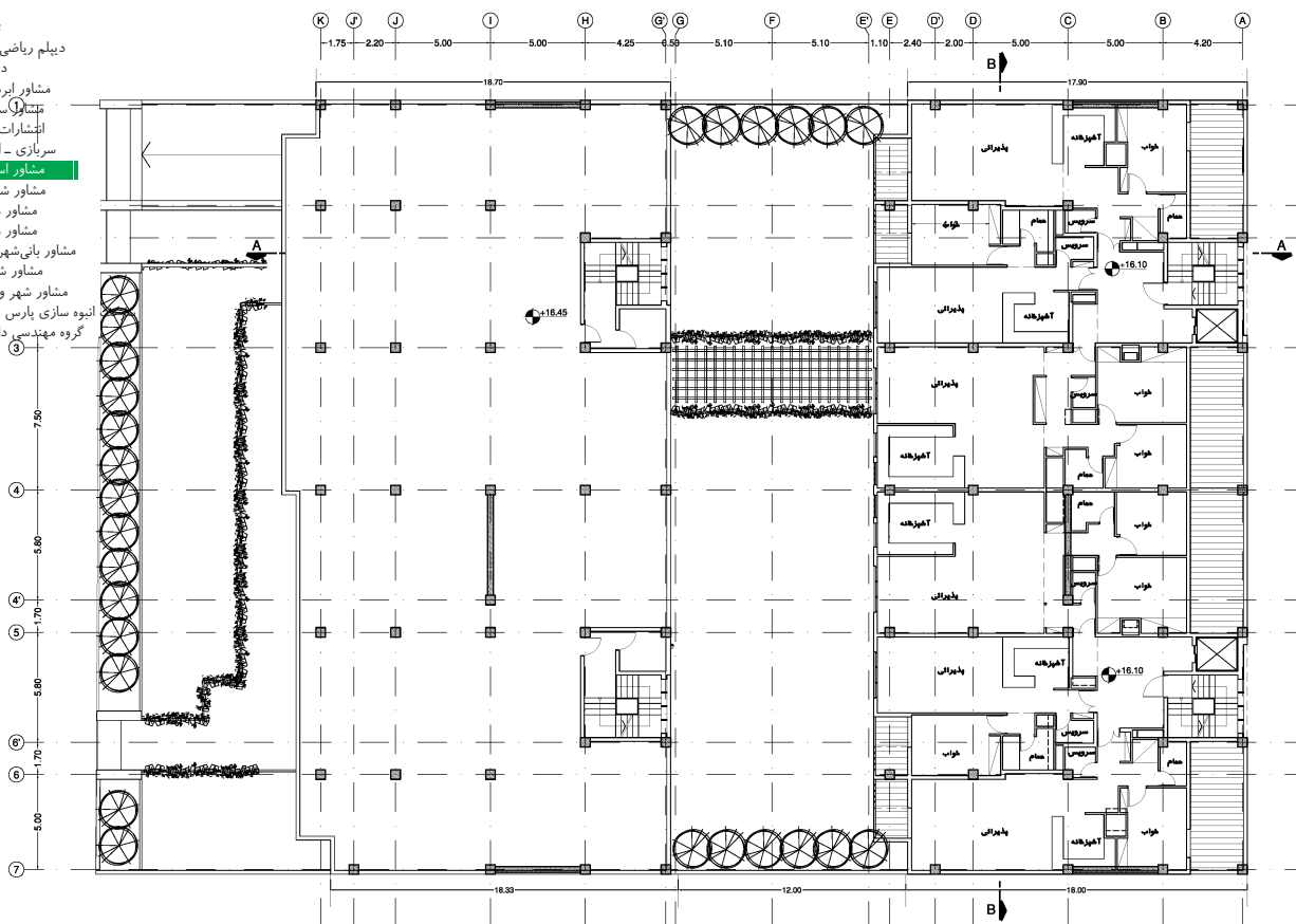
پلان طبقه پنجم
